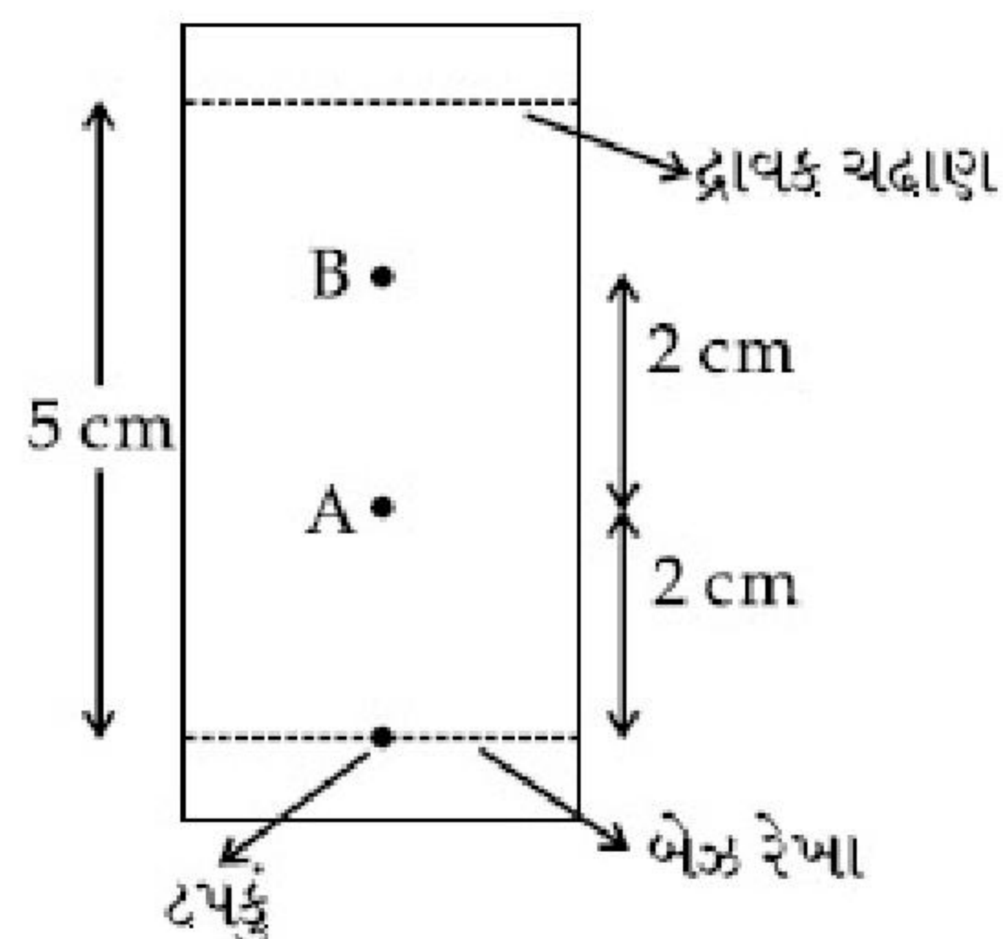
આકૃતિ : સંયોજનો A અને B માટે પેપર ક્રોમેટોગ્રાફી
