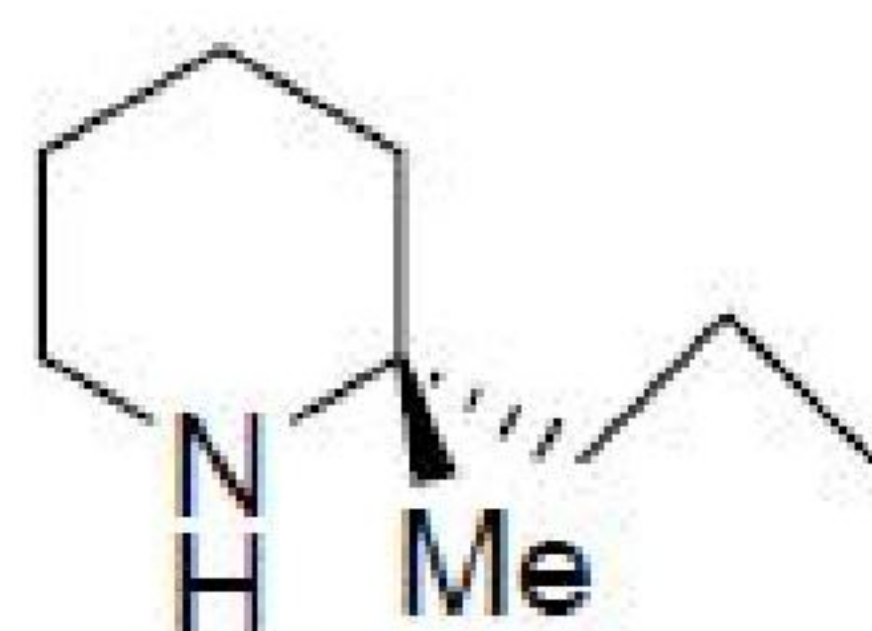
Coniine
