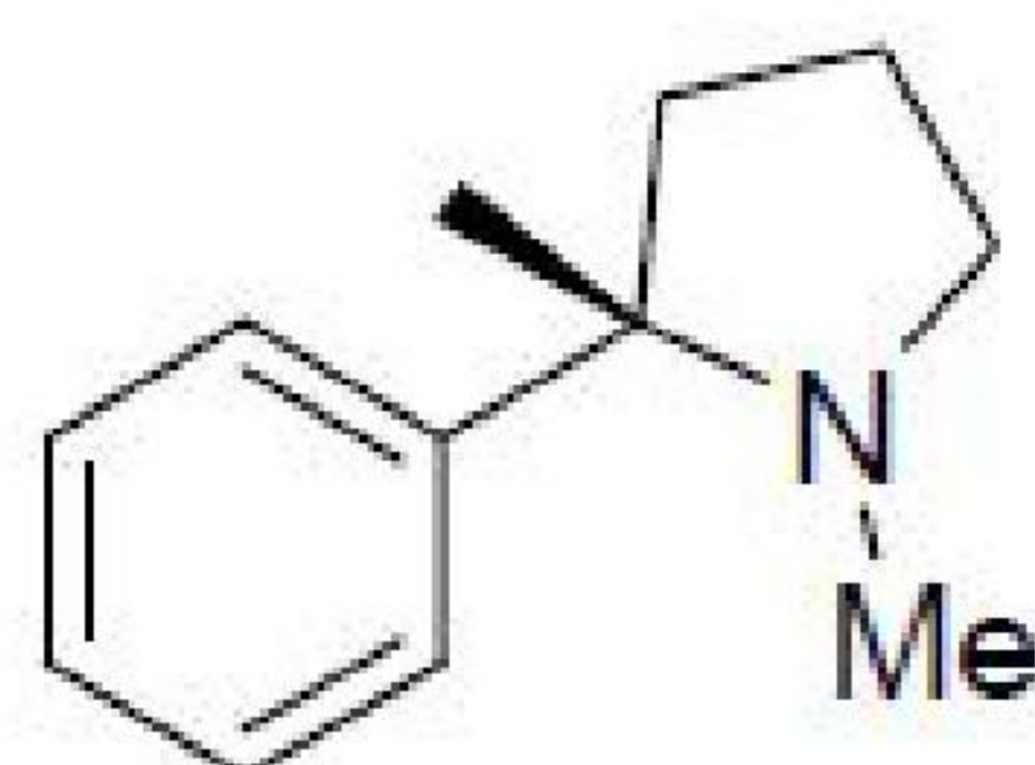
Nicotine
